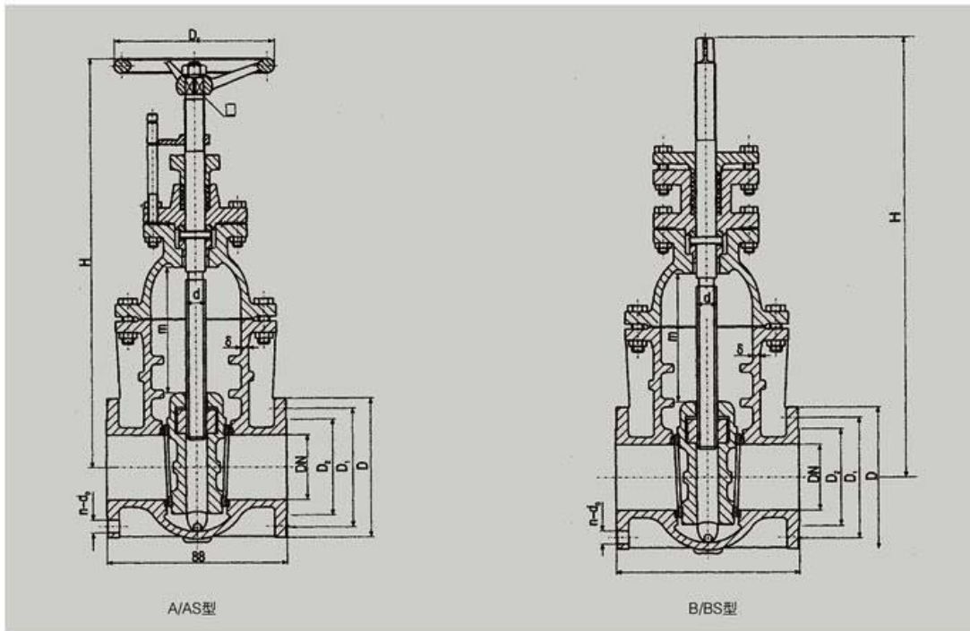
主要零部件材质 Materials of Main Parts
